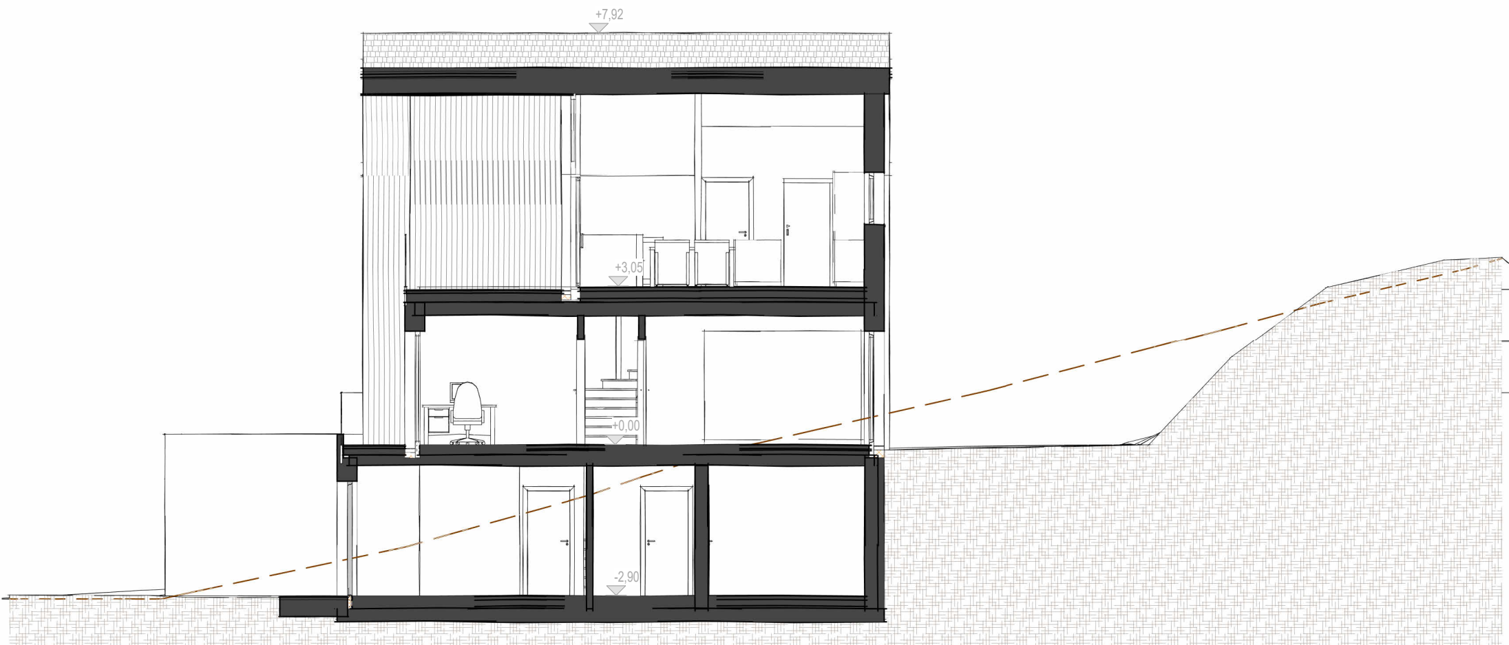
SCHNITT A-A M 1:100
