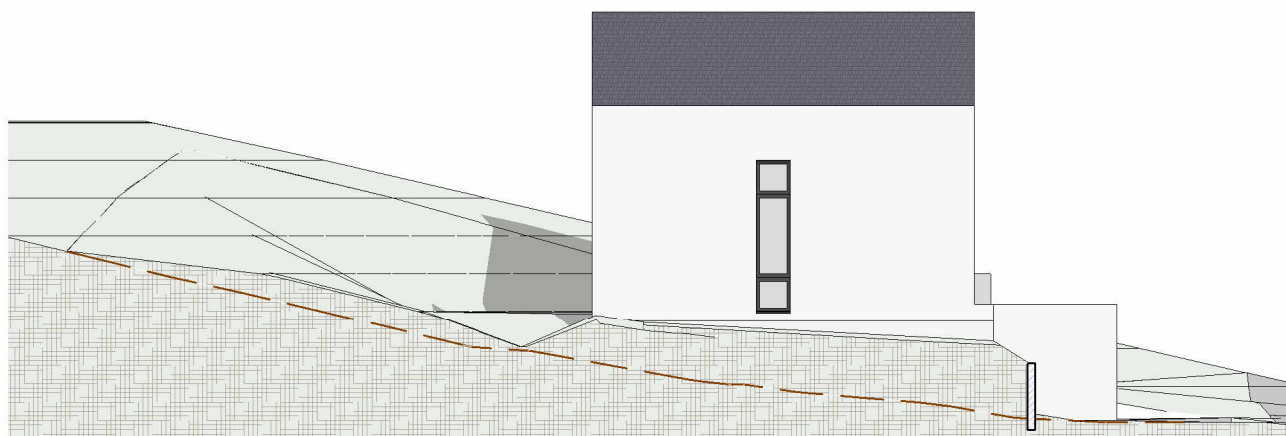
WESTANSICHT
